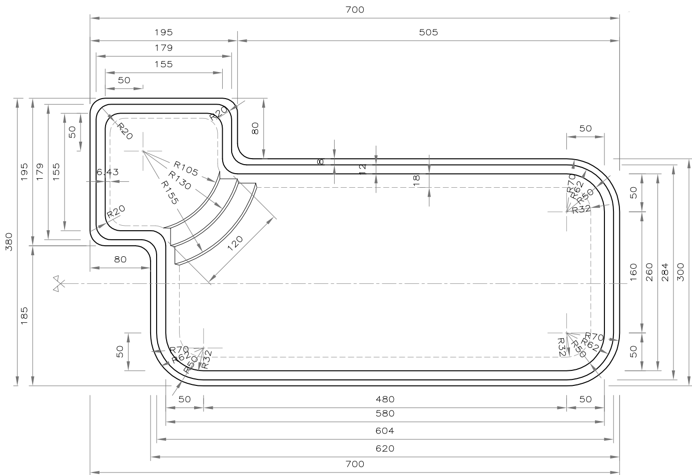
Vista Superior Escala 1/50
