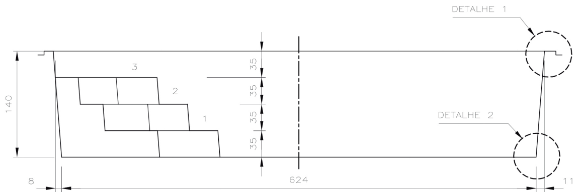
Corte Longitudinal Escala 1/50
